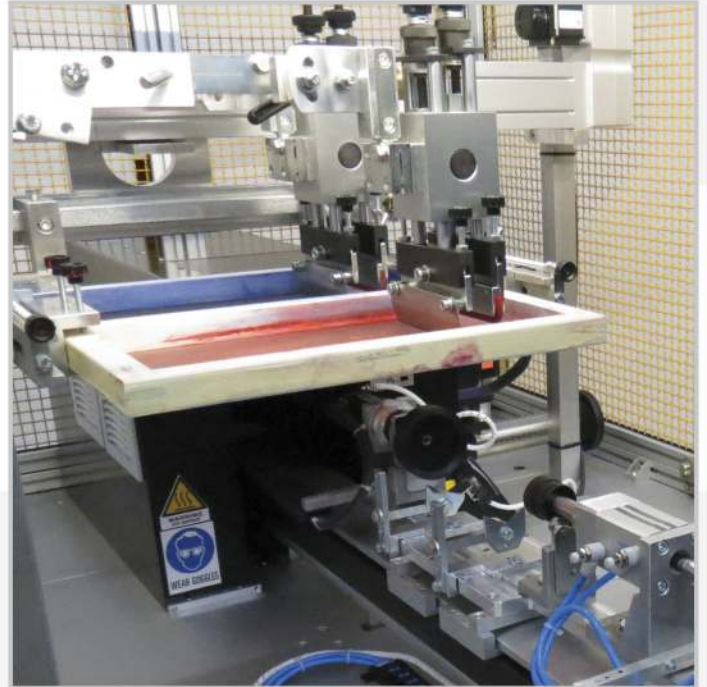
DOPPIO TELAIO DI STAMPA DOUBLE SCREEN
